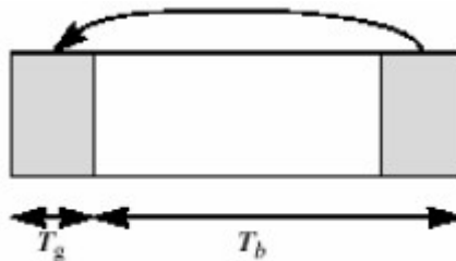
Рис. 4.14. OFDM-символ с циклическим префиксом
