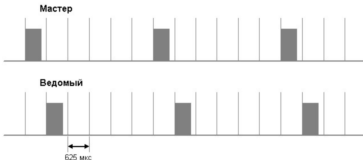
Рис. 4.4. Передача пакетов при синхронном соединении
